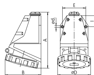
EZH 12543
