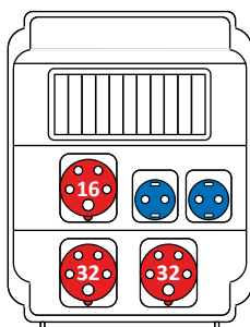
EDS11 2-2/3-5 32/16
