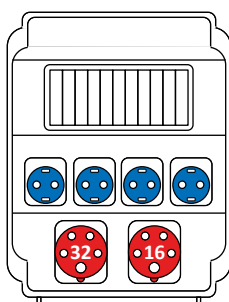
EDS11 4-2/2-5 16/32
