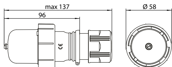
EEVG 16
