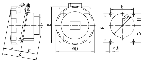
EEH 1632
