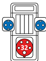
EDS4m 2-2/1-5 32
