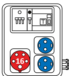
EDS8 RCD 2-2/1-5 16
