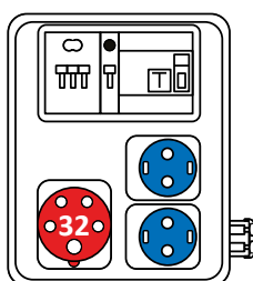
EDS8 RCD 2-2/1-5 32
